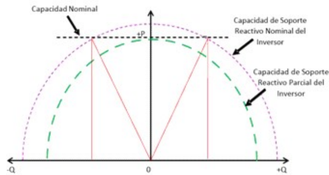
Figura No 6. Ejemplo Curva de Capacidad del Aerogenerador
