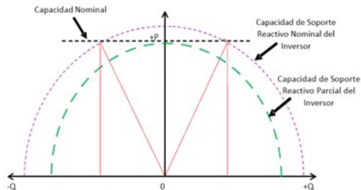
Figura No 3. Ejemplo de Curva de Capabilidad de Inversor
