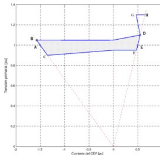
Figura No 2 Ejemplo de Curva de Operación de SVC
