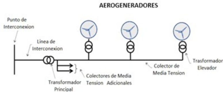
Figura No 2. Ejemplo de Diagrama Unifilar Detallado
