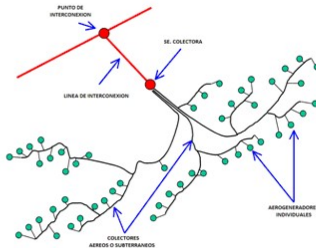
Figura No 3. Ejemplo de Diagrama Topológico del Parque Eólico
