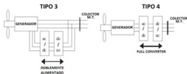
Figura No 4. Ejemplos de Tipos de Aerogeneradores
