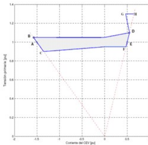
Figura No 5 Ejemplo de Curva de Operación de SVC
