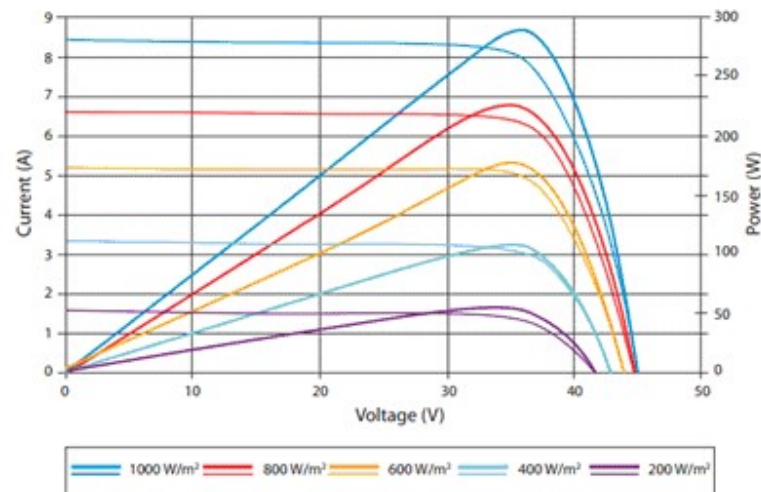
Figura 4. Ejemplo de Curva de I-V, P-V.
