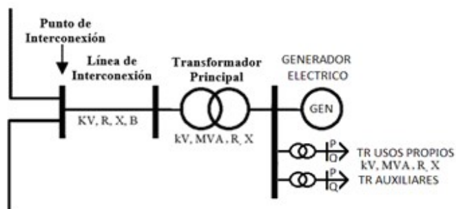
Figura No 2. Ejemplo de Diagrama Unifilar Simplificado
