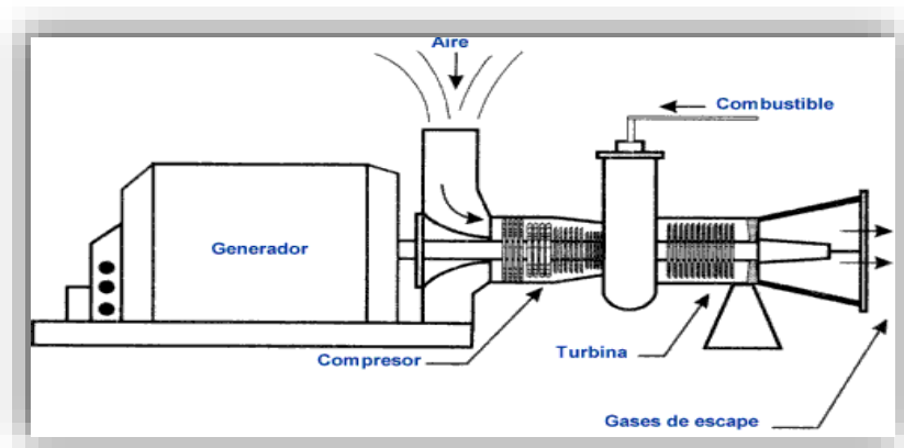
Figura 3. Ciclo de la Turbina de Gas 2 .
