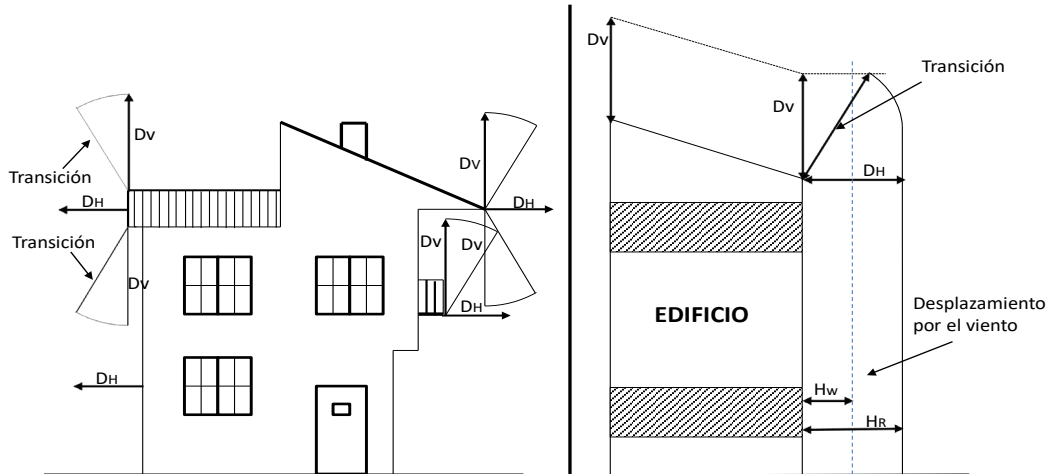
Figura 3. Distancias de seguridad a edificaciones
