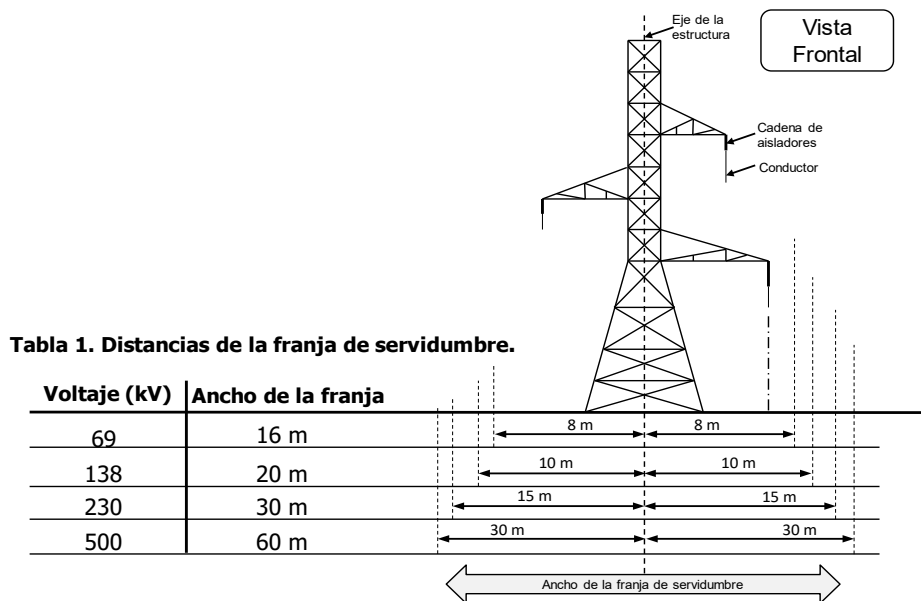
Figura 1. Ancho de las franjas de servidumbre.
